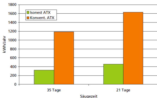
Energieverbrauch pro Ferkelnest und Jahr
